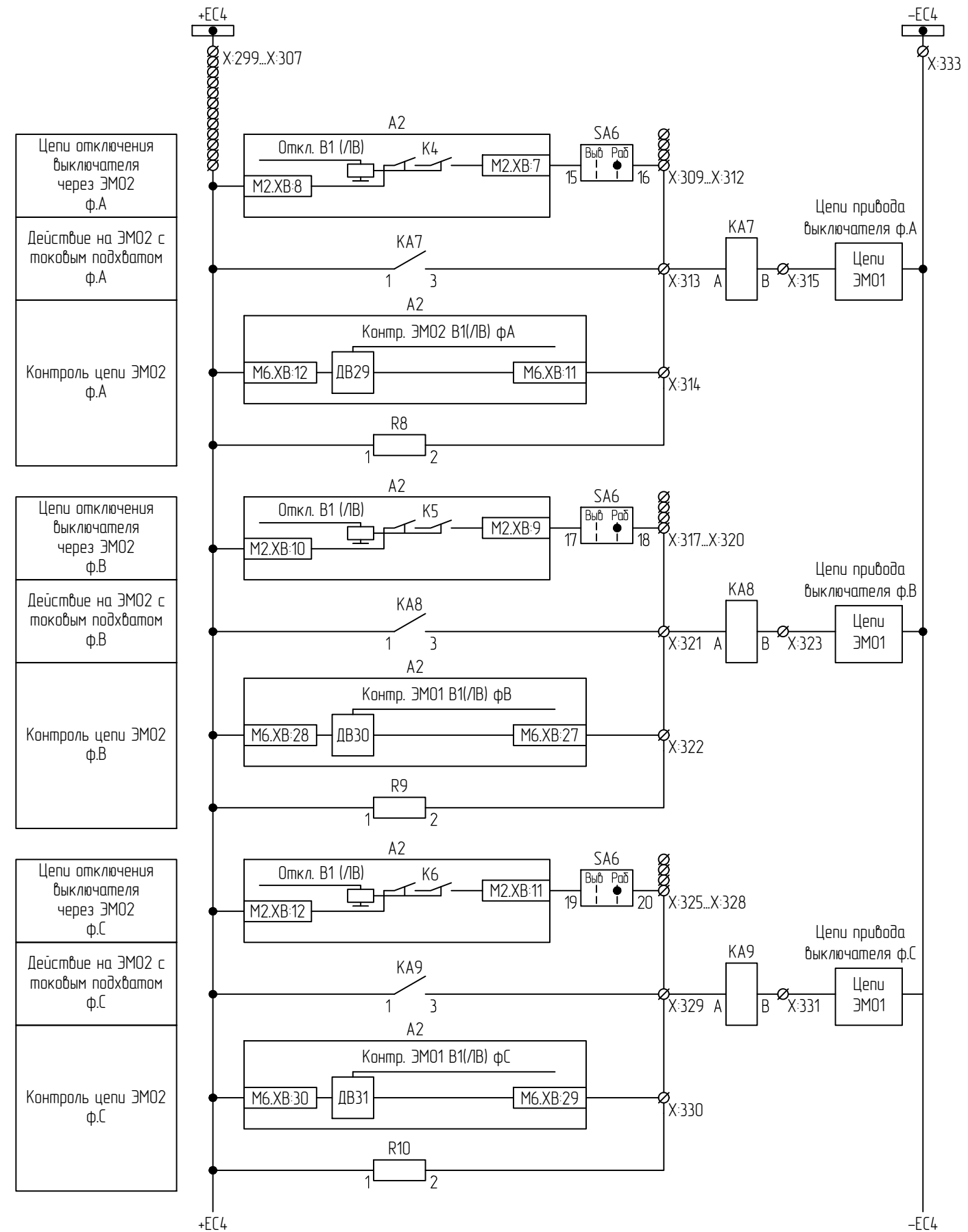
Цепи ЭМ02
