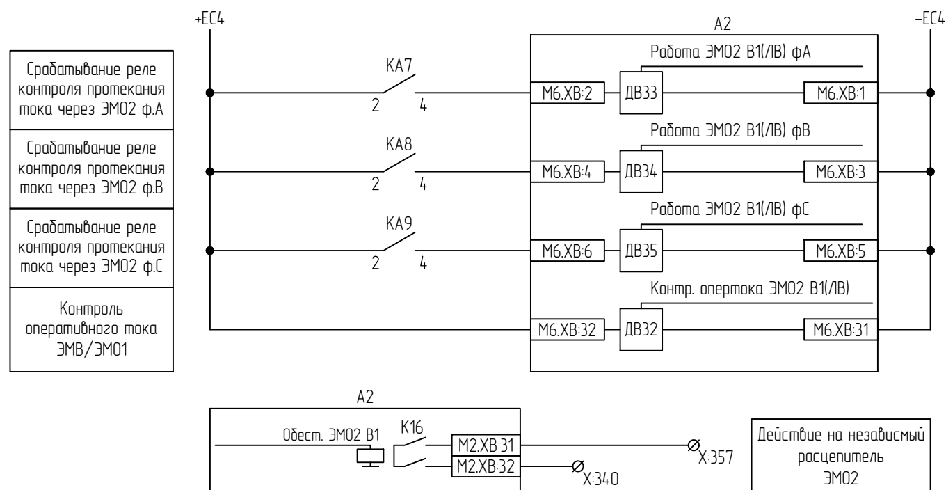
Цепи ЭМ02
